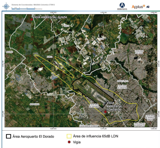
Panorama de las estaciones de monitoreo inteligente de ruido y Vigas Ambientales del Aeropuerto Internacional. Fuente Aerocivil 2025
